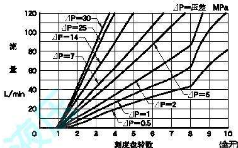
开度—流量特性
