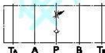
详细液压图形符号
