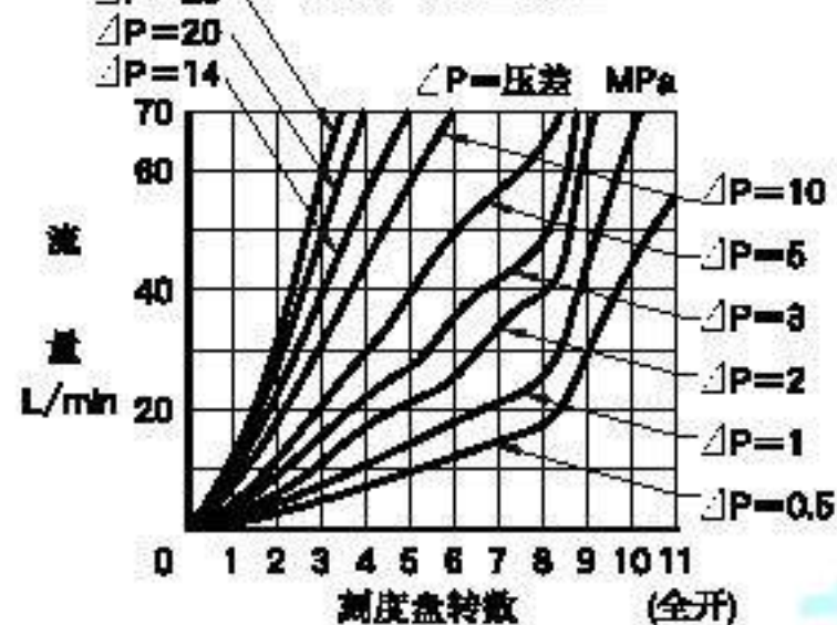
开度-流量特性
