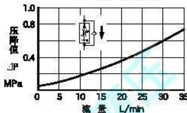
自由流压降特性
