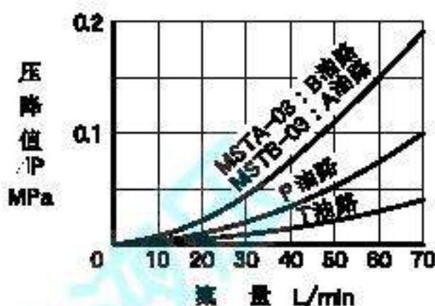
各油路压降特性
