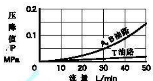
各油路压降特性
