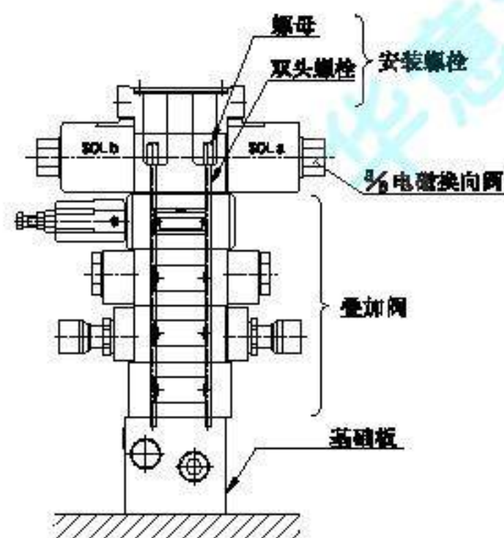
03系列叠加阀装配例
