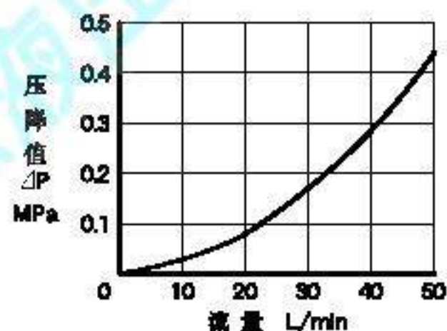
阀芯全开时的压降特性 (P油路)
