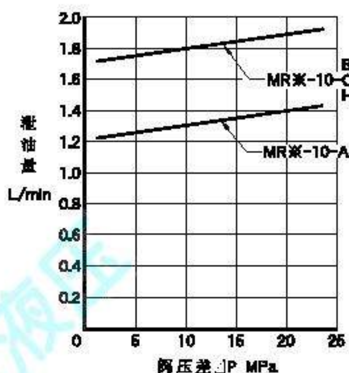
泄油量特性
