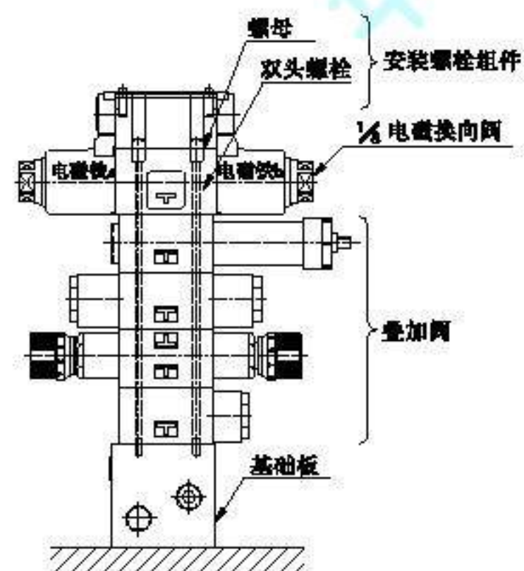
01系列叠加阀装配例
