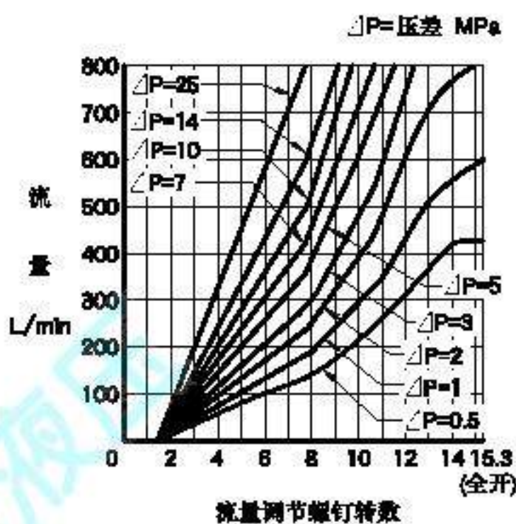
开度—流量特性
