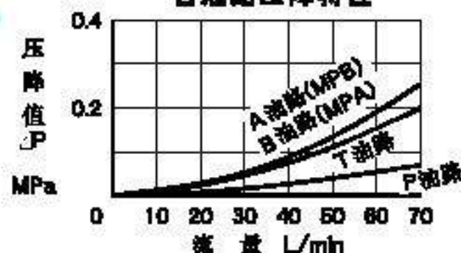
自由流压降特性
