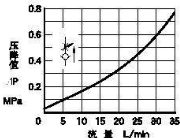
各油路压降特性
