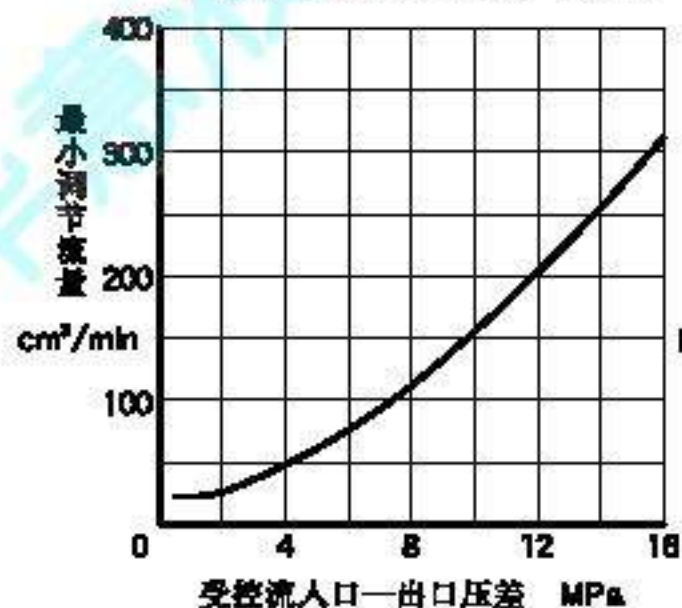
压力—最小调节流量特性
