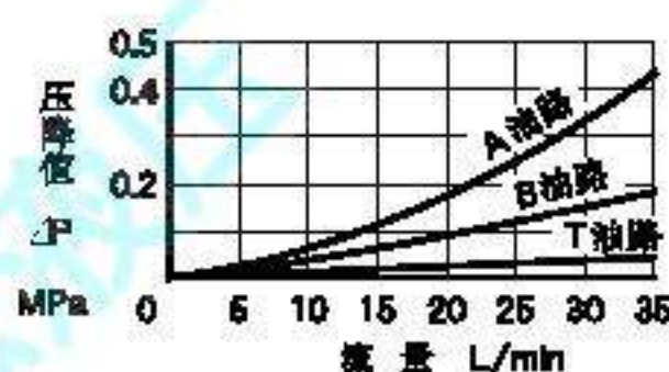
各油路压降特性
