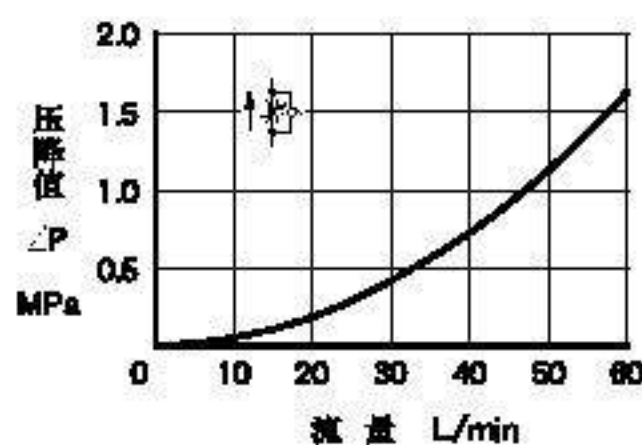
节流阀全开时的压降特性
