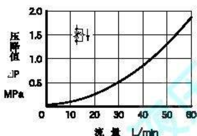
自由流压降特性
