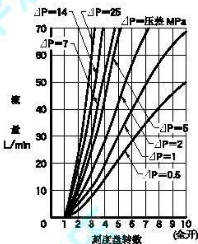
开度—流量特性
