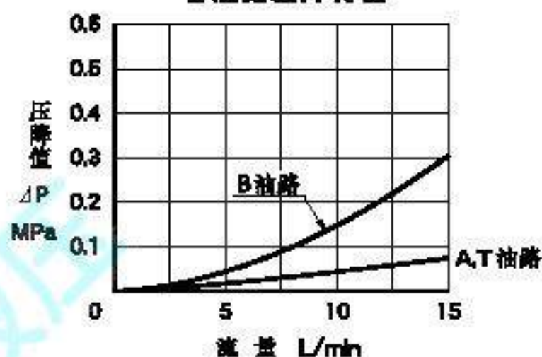
各油路压降特性
