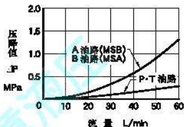
各油路压降特性
