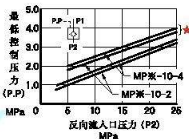
最低控制压力特性
