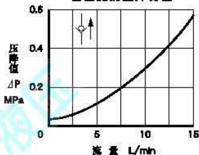
自由流的压降特性
