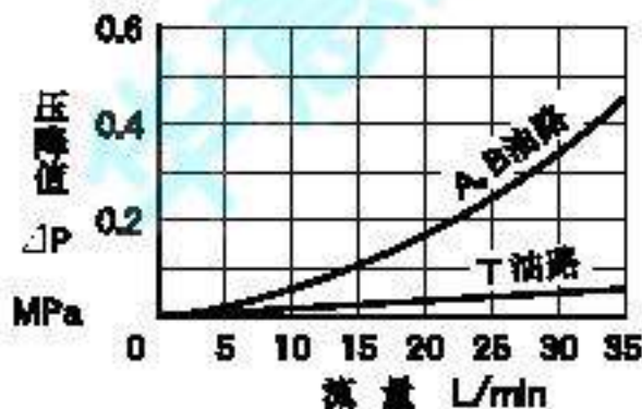
各油路压降特性 MHA-01
