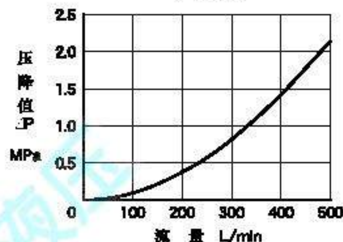
阀芯全开时的压降特性 (P油路)
