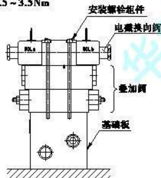
螺栓标记
