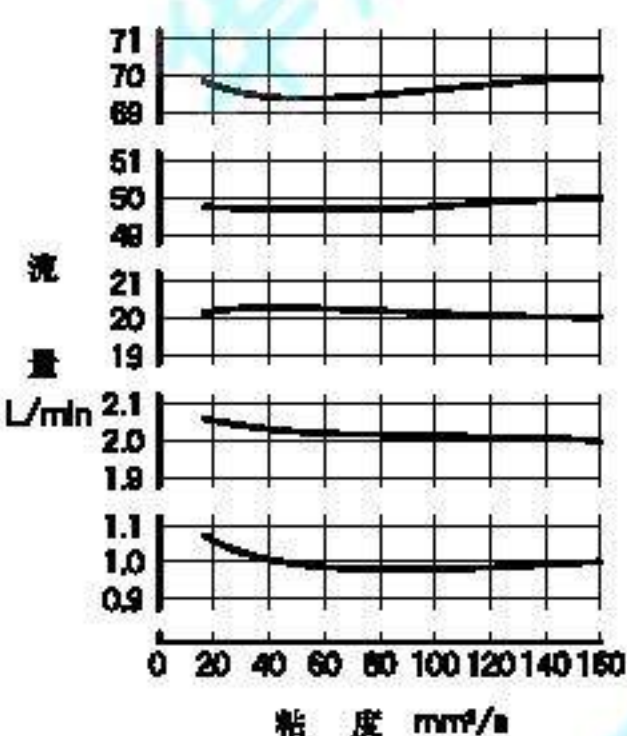
粘度—流量特性
