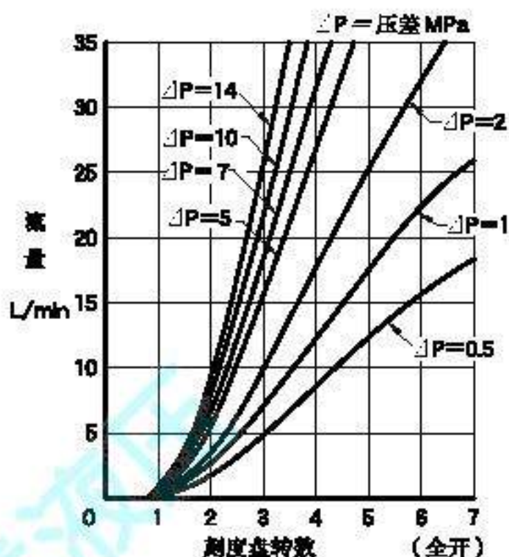
关闭—流量特性
