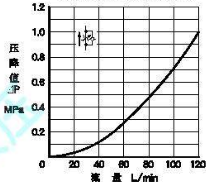
节流阀全开时的压降特性
