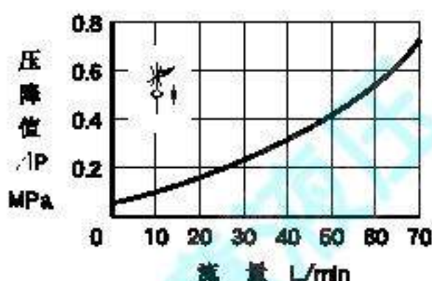
节流阀全开时的压降特性
