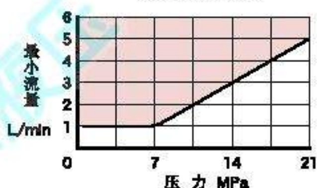
压降特性
