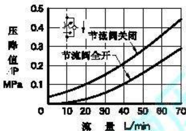
自由流压降特性
