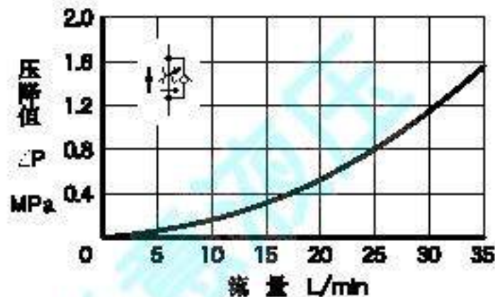
节流阀全开时的压降特性
