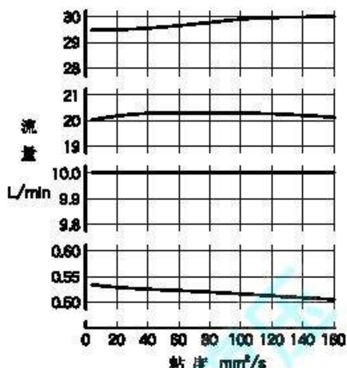
粘度—流量特性
