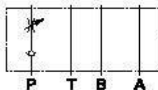
JIS液压图形符号
