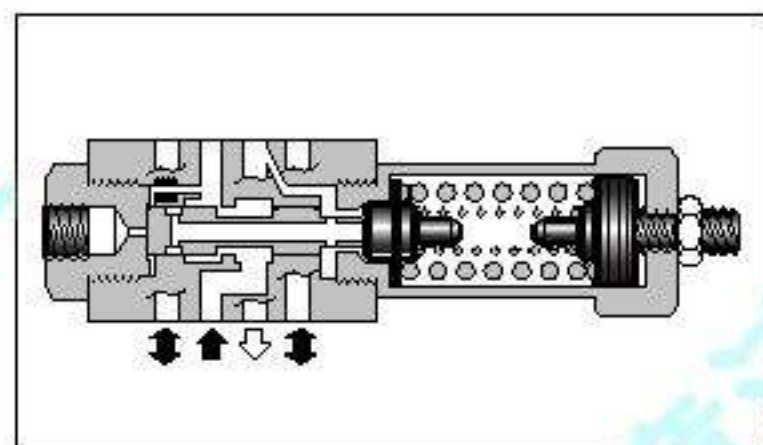
JIS液压图形符号
