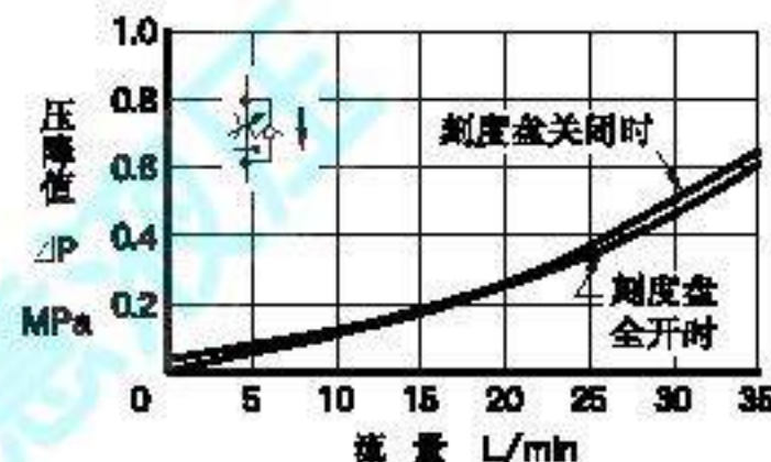
自由流—压力下降特性
