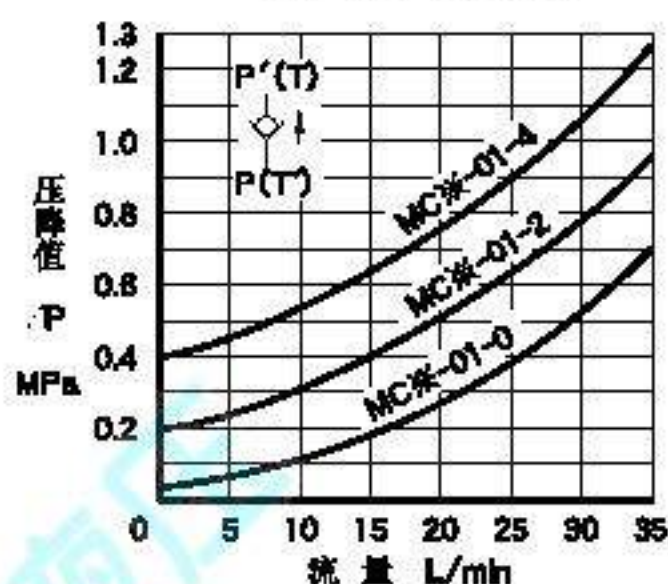
自由流压降特性
