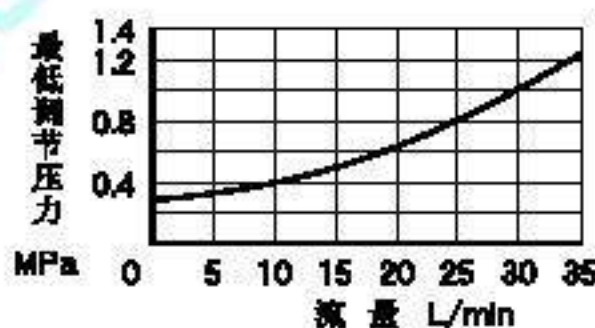
最低调节压力特性 MHP/MHA-01
