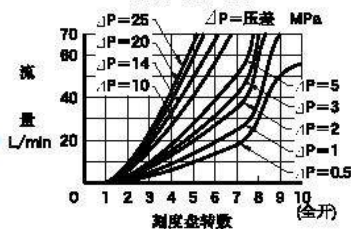
开度-流量特性
