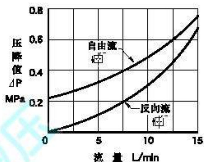
自由流/反向流—压降特性
