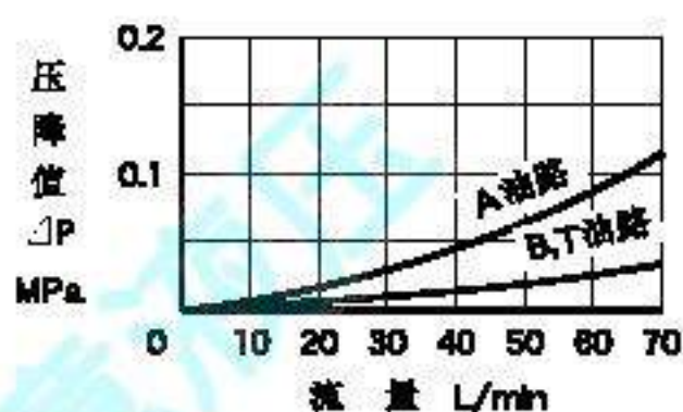
各油路压降特性
