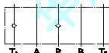
详细液压图形符号
