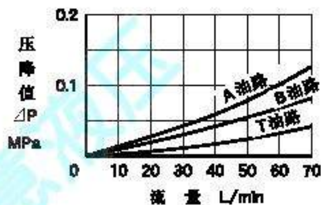
各油路压降特性
