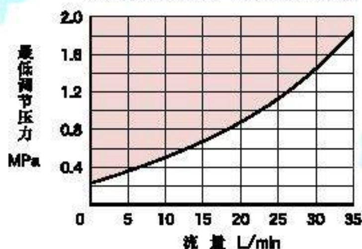
最低调节压力—最大流量特性
