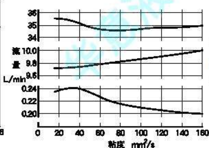
粘度—流量特性
