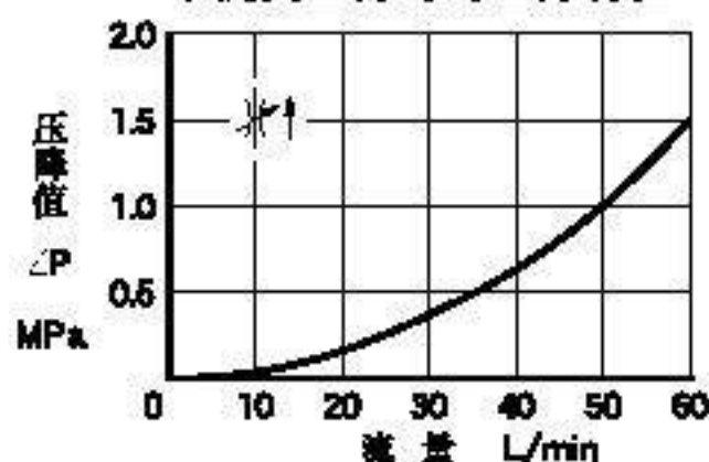
节流阀全开时的压降特性
