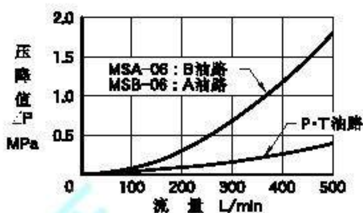
各油路压降特性
