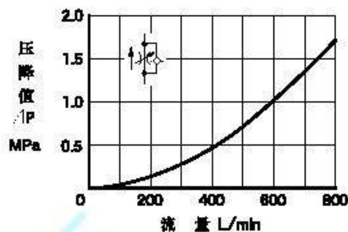
节流阀全开时的压降特性
