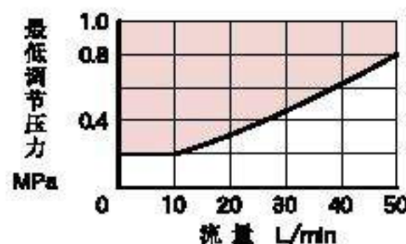
最低调节压力—最大流量特性
