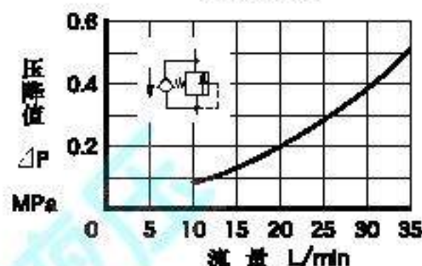
自由流压降特性 MHA-01
