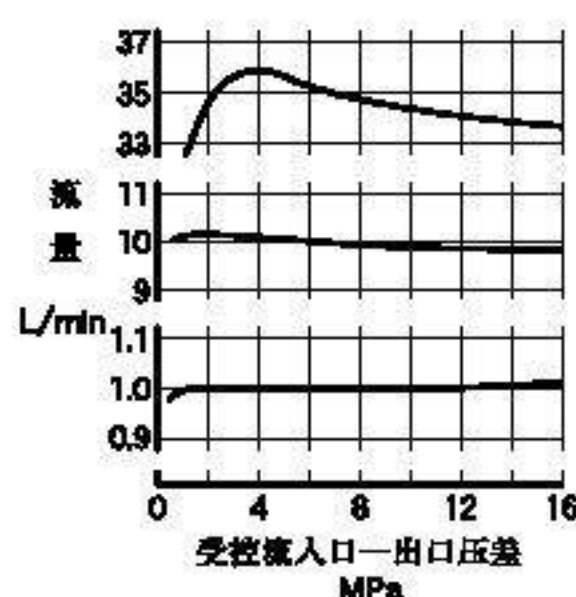
压力流量特性
