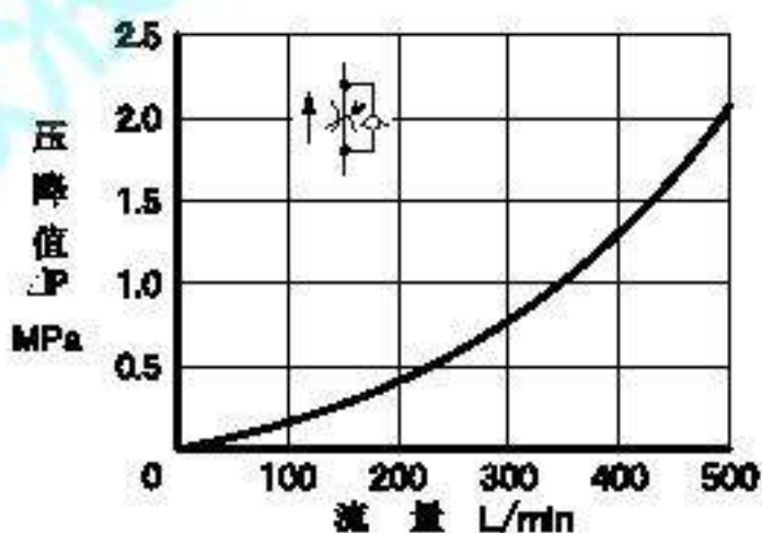
节流阀全开时的压降特性
