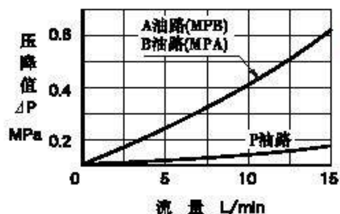
各油路压降特性
