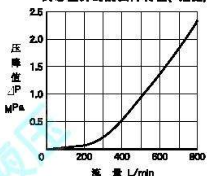
阀芯全开时的压降特性(P油路)
