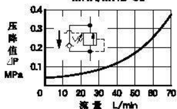
自由流压降特性 MHA/MHB-03
