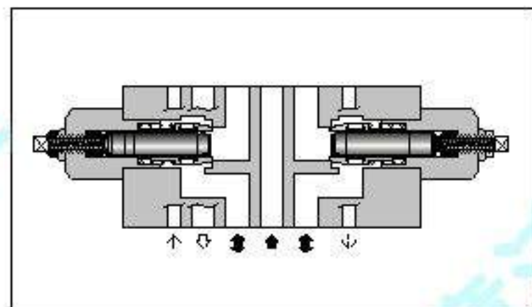
JIS液压图形符号
