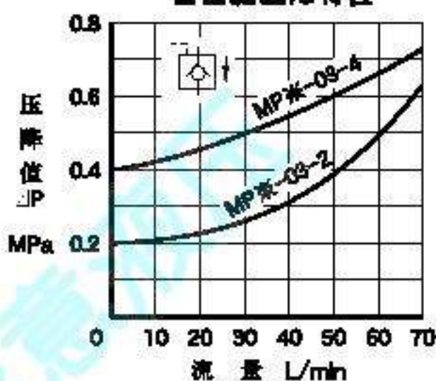
自由流压降特性
