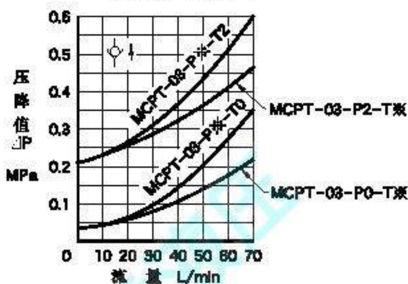
自由流压降特性
