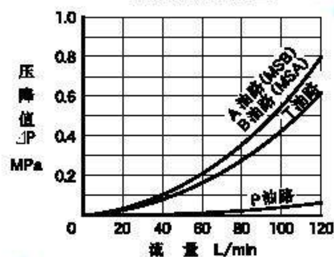
自由流压降特性
