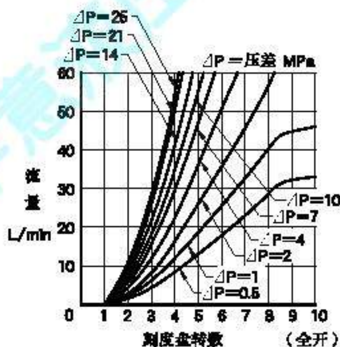
开度—流量特性
