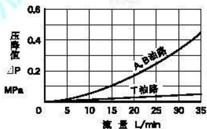
压降特性
