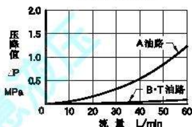
各油路压降特性
