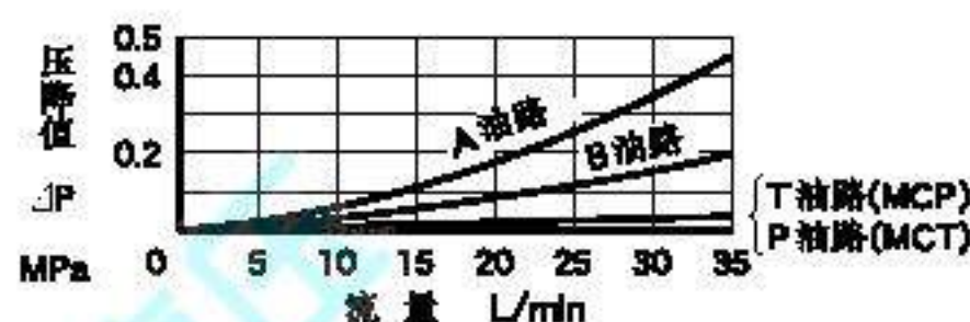
各油路压降特性
