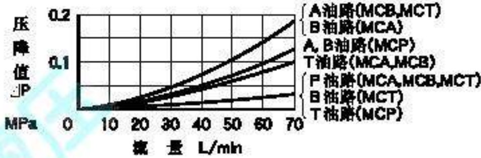
各油路压降特性
