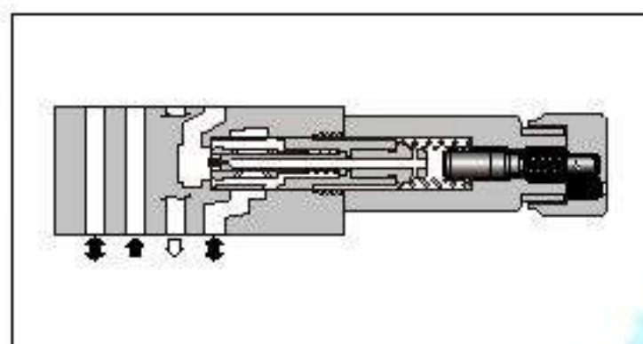
JIS液压图形符号
