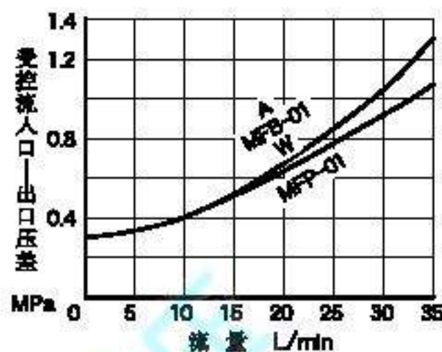
所需最低压差特性
