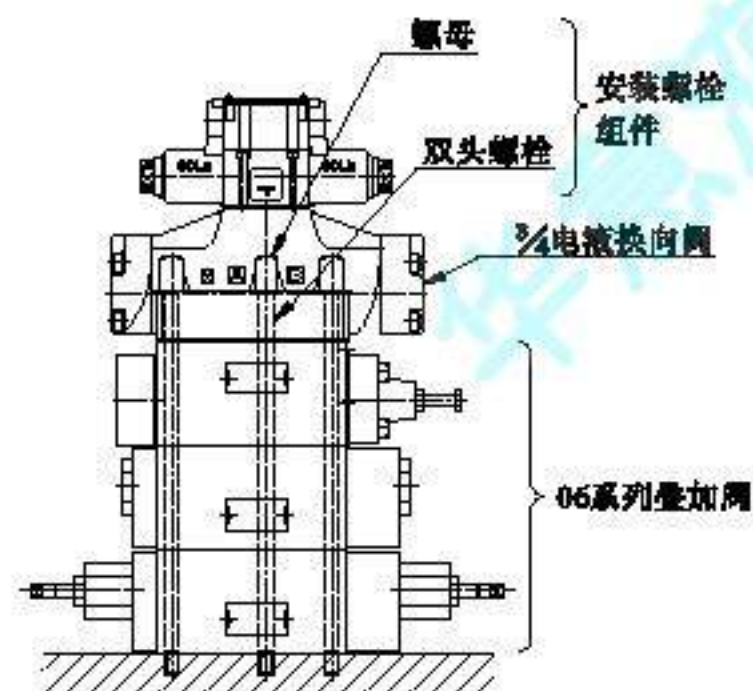
06系列叠加阀装配例
