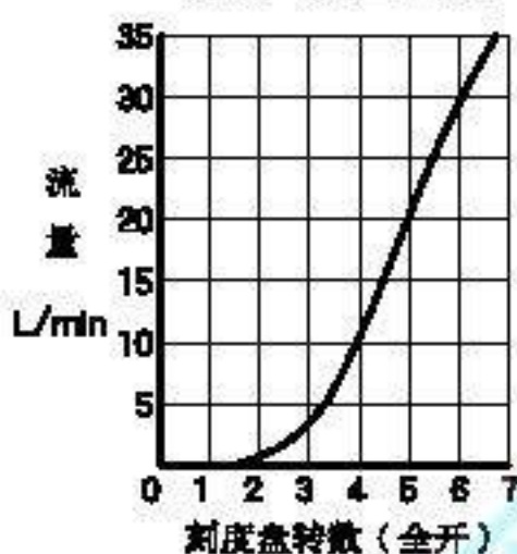
开度—流量特性
