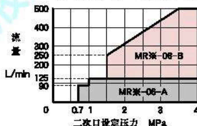
二次口设定压力-最大流量特性
