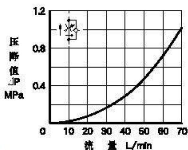
节流阀全开时的压降特性
