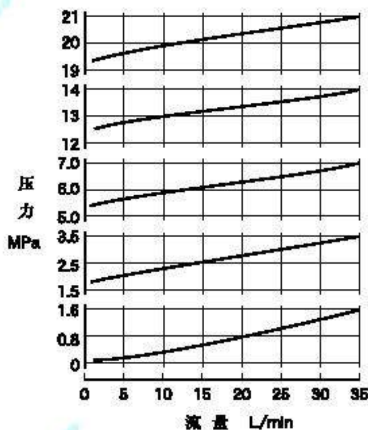
压力—流量特性
