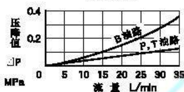
各油路压降特性 MHA-01
