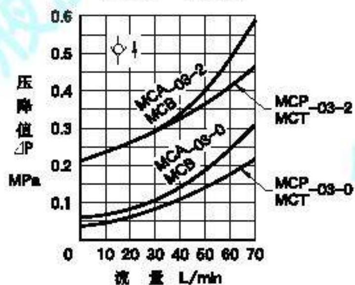
自由流压降特性
