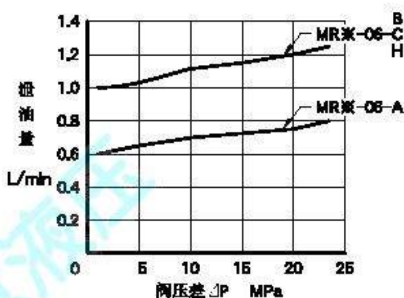
泄油量特性
