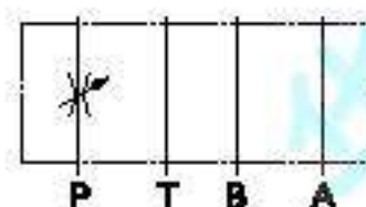
JIS液压图形符号
