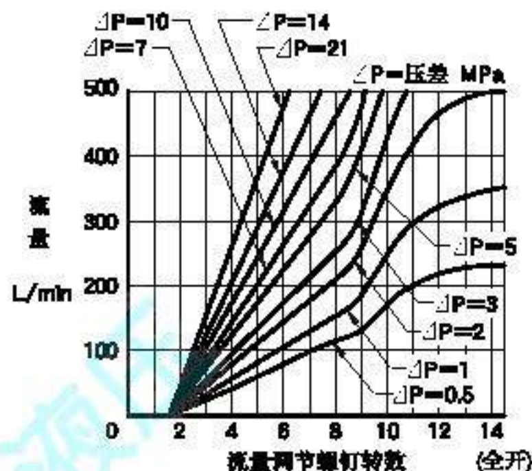
开度—流量特性
