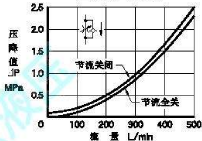
自由流压降特性
