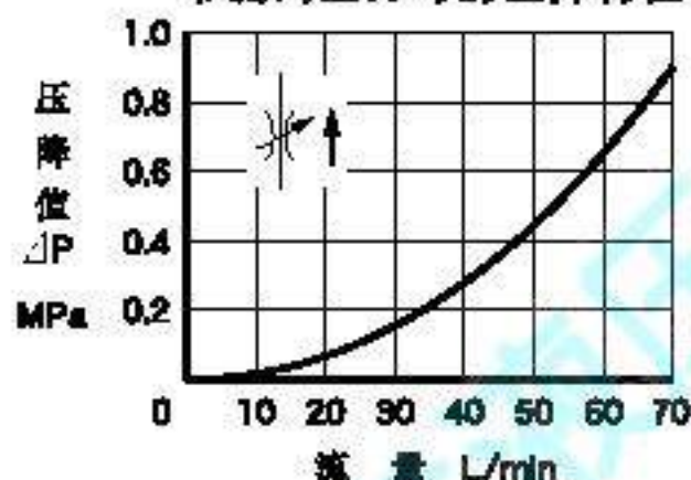
节流阀全开时的压降特性
