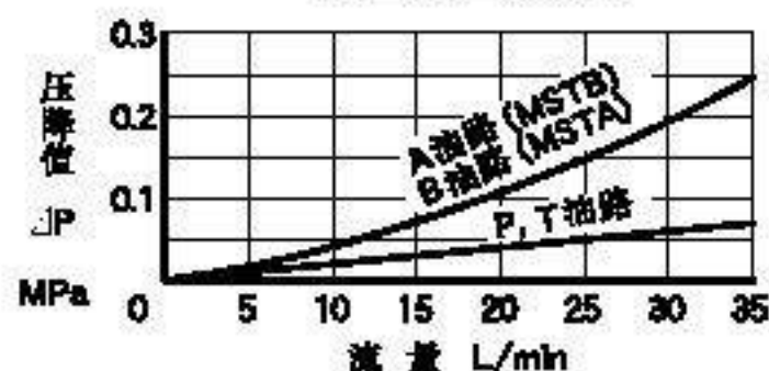
各油路压降特性
