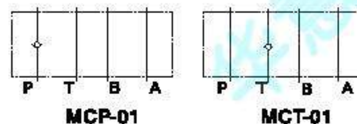
JIS液压图形符号
