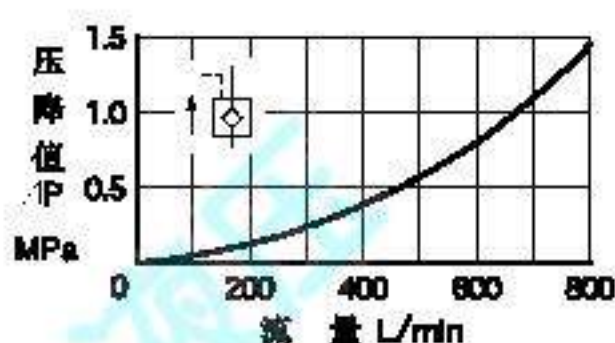
反向流压降特性
