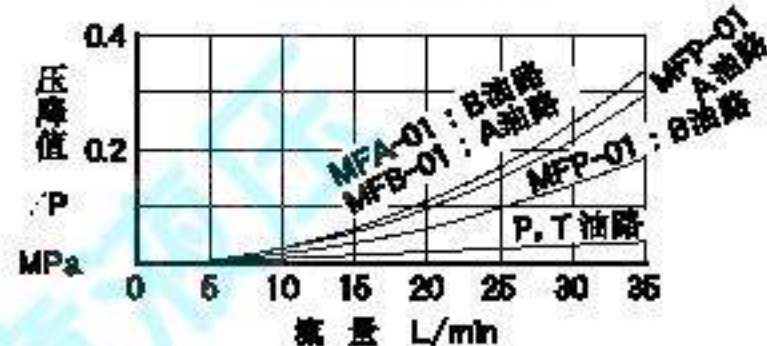
各油路压降特性
