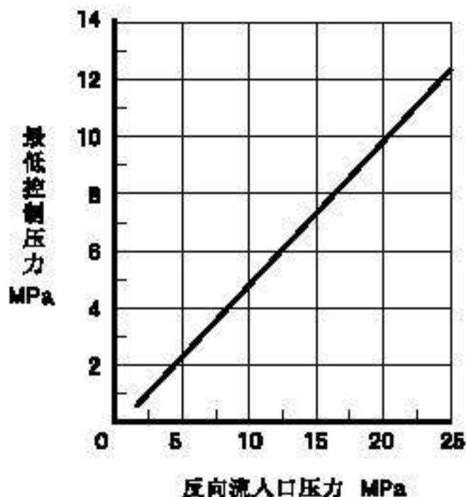
最低控制压力特性
