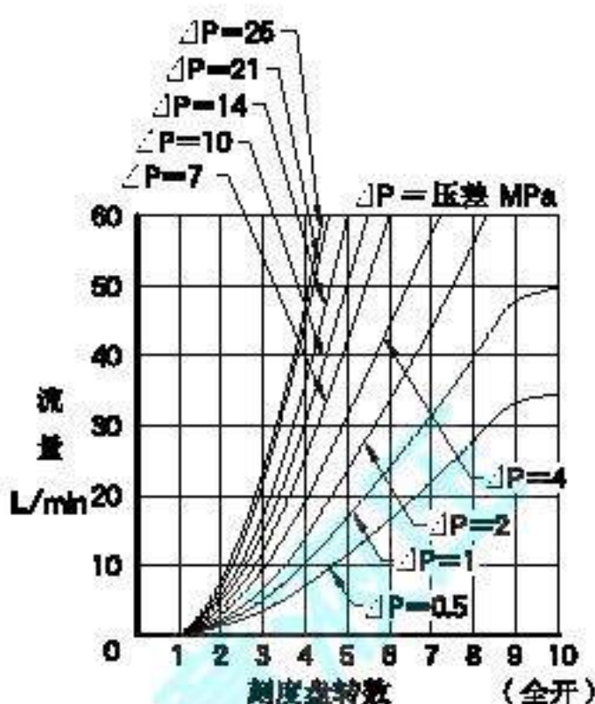
开度—流量特性
