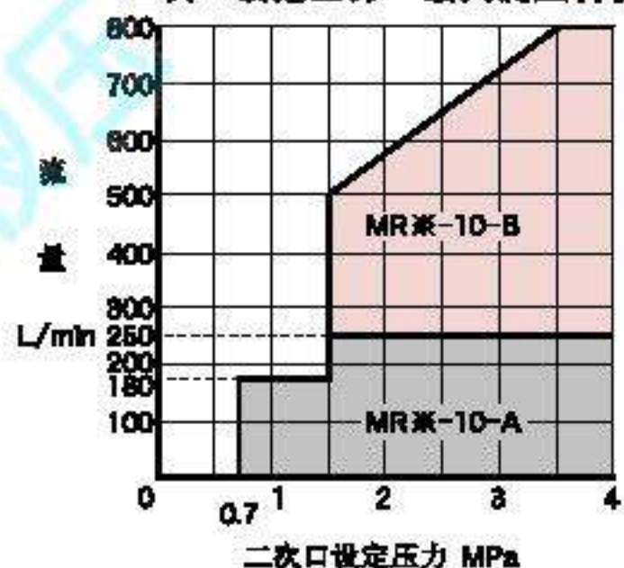
二次口设定压力—最大流量特性
